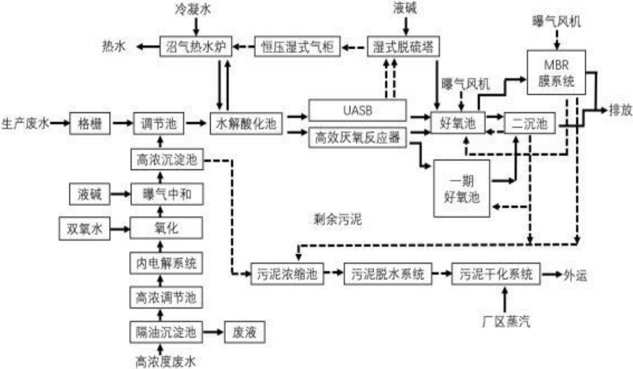
图 4.1-1 污水处理工艺流程图
