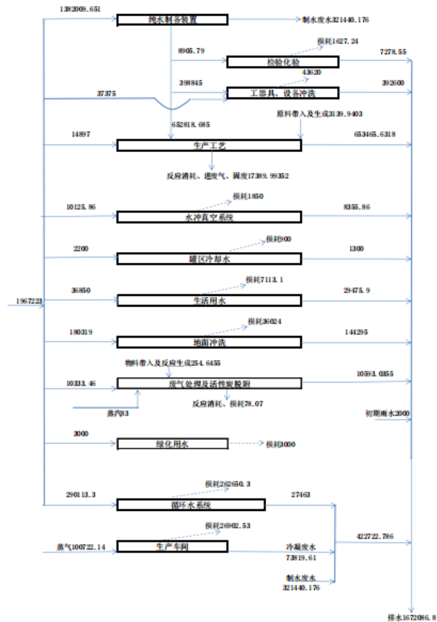
图 3.5-1 项目全厂水平衡图 (t/a)
